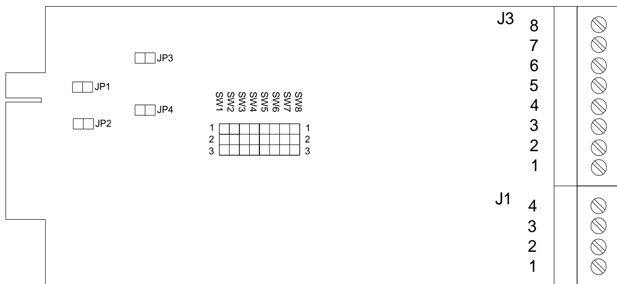
Figura 1: Allocazione dei punti di settaggio e delle morsettiere
